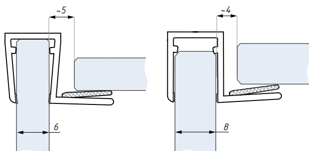
do szkła 6 mm
