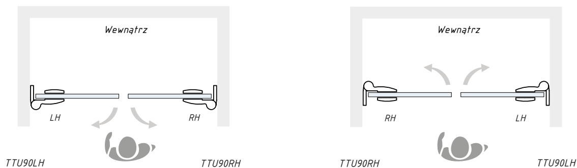
Zawiasy ścianna - szkło
