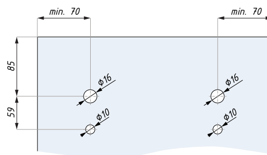
Przygotowanie szkła, panel przesuwny
