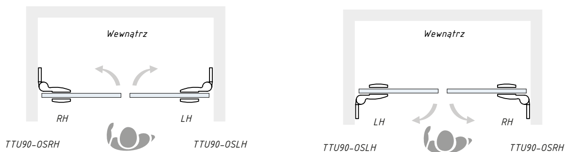
Zawiasy z mocowaniem bocznym ścianna - szkło
