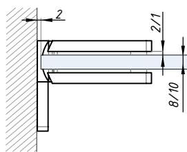
Przygotowanie szkła do szczeliny 2 mm
