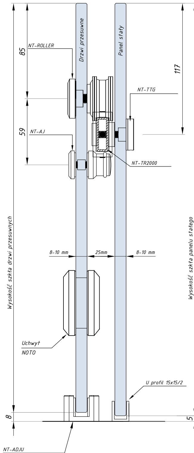
Wariant z dwoma wózkami i zabezpieczeniem ANTIJUMP
