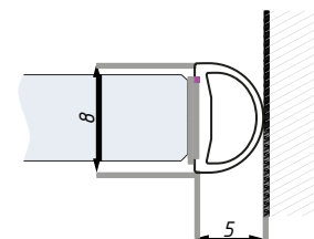
montáž na zed'
