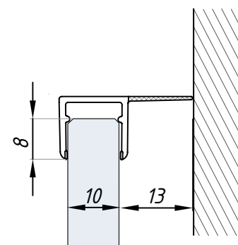
Těsnění SDEN 8x10 montáž na sklo 10 mm
