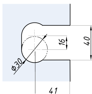
Příprava skla pro sklo 8 mm s těsněním ABE6-8
