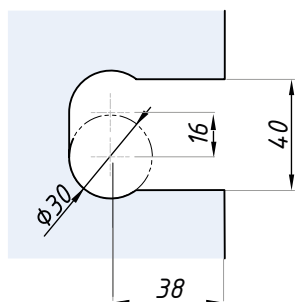
Příprava skla pro sklo 10 mm s těsněním ABE10
