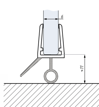
Těsnění DOE 6x8 montáž na sklo 6 mm
