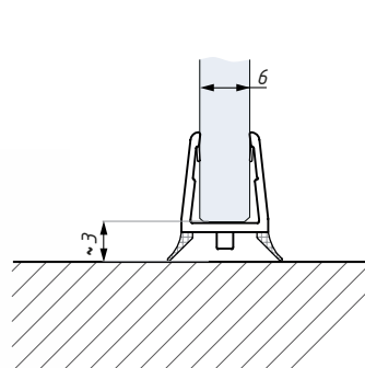
Těsnění GCE 6x8 montáž na sklo 6 mm
