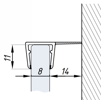
Těsnění SDEN 8-10 montáž na sklo 8 mm
