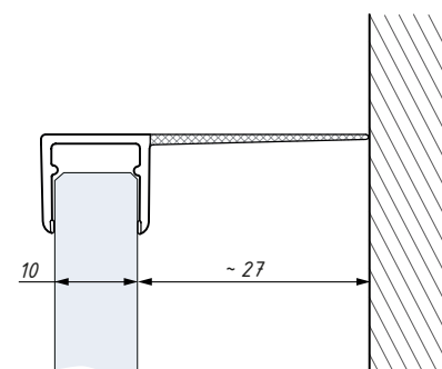
Těsnění SDE 8-10 montáž na sklo 10 mm
