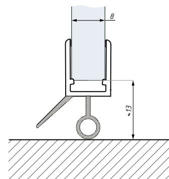
Těsnění DOE 6x8 montáž na sklo 8 mm
