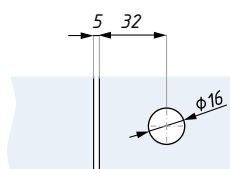
Příprava skla: varianta sklo - sklo
