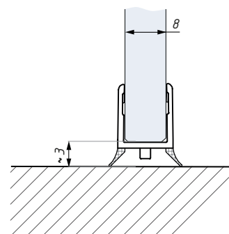
Těsnění GCE 6x8 montáž na sklo 8 mm
