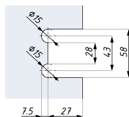
Příprava skla pro mezeru 0-5 mm
