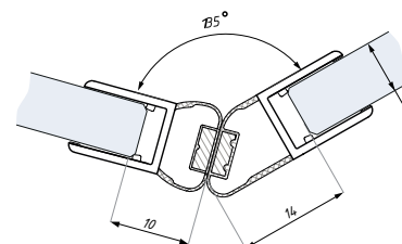
Těsnění PMSE 6x8 montáž na sklo 8 mm
