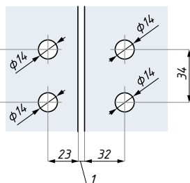
Příprava skla 8 mm
