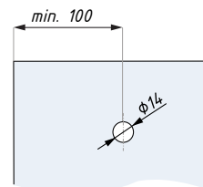
Příprava skla, posuvný panel
