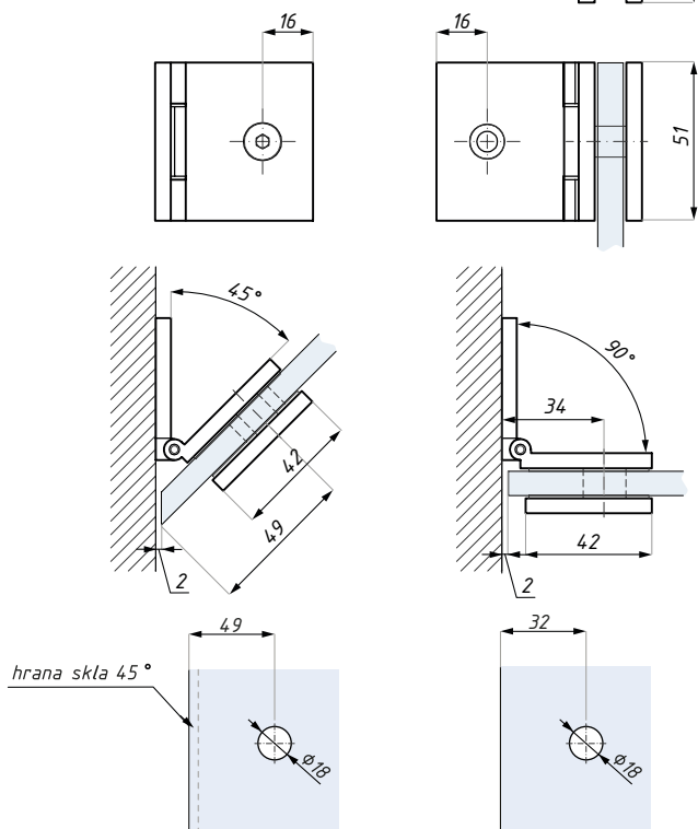
Příprava skla pro nastavení 45°
