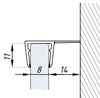
Těsnění SDEN 8x10 montáž na sklo 8 mm
