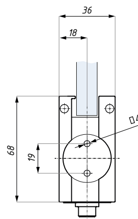
Samozavírací dolní závěs
