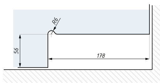
Příprava skla pro samozavírací závěs
