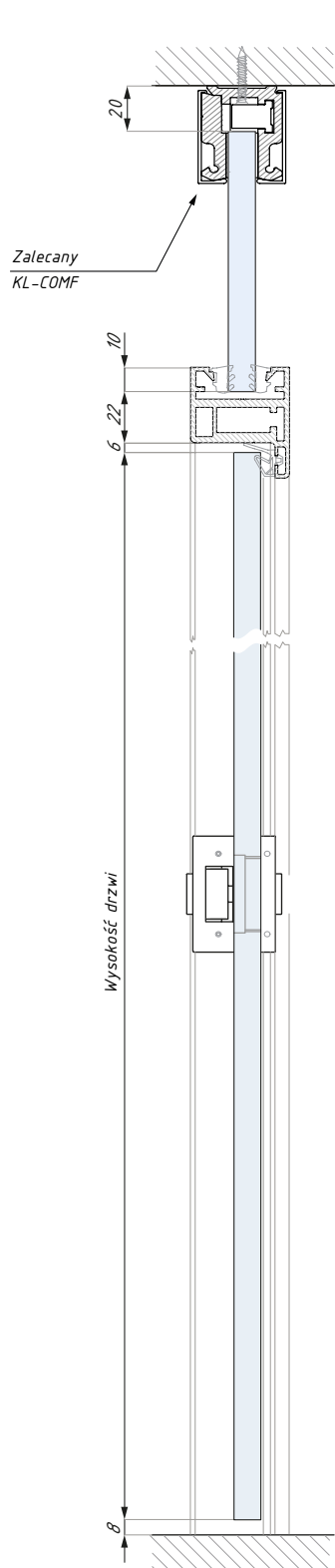
Profil drzwiowy PAL-H z naświetłem
