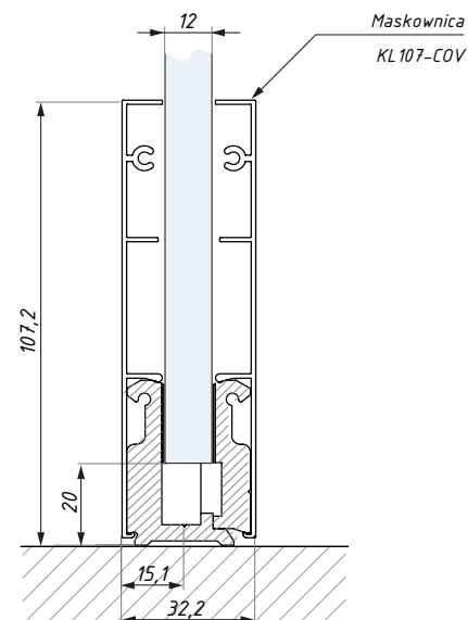
Profil KL-ECON 12 (szkło 12 mm)
