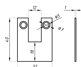
KL41EC-12 Do szkła 12 mm
