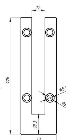
KL107EC-12 Do szkła 12 mm
