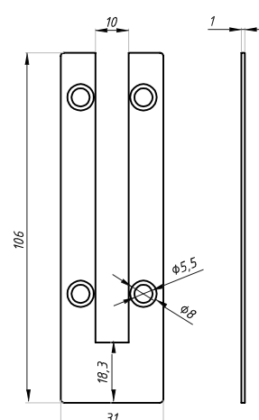
KL107EC-10 Do szkła 8 a 10 mm
