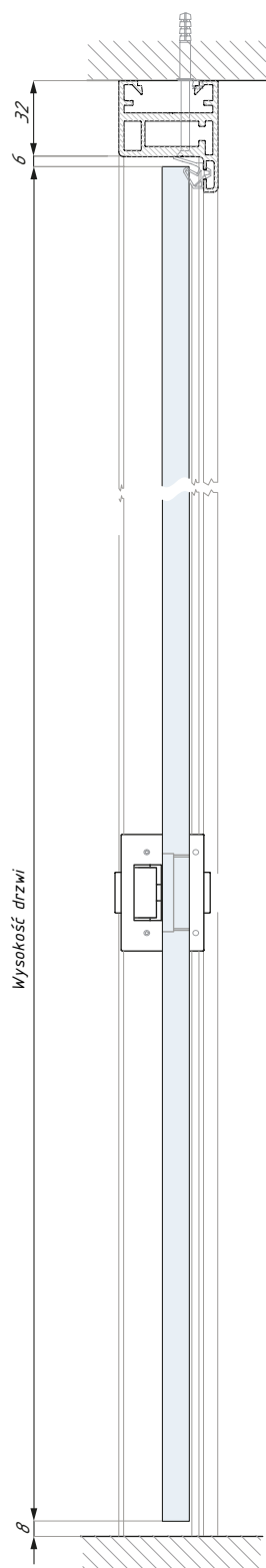
Profil drzwiowy PAL-H bez naświetła
