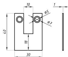
KL41EC-10 Do szkła 8 a 10 mm
