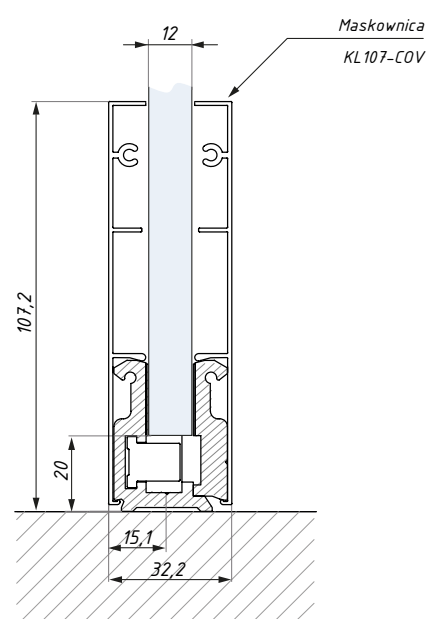
Profil KL-COMF 12 (skło 12 mm)
