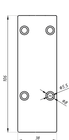
KL107EC-16 Do szkła 16,76 a 17,52 mm
