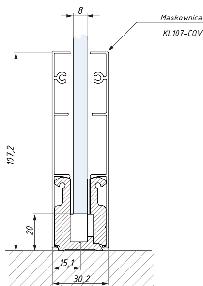
Profil KL-ECON 8 (szkło 8 mm)
