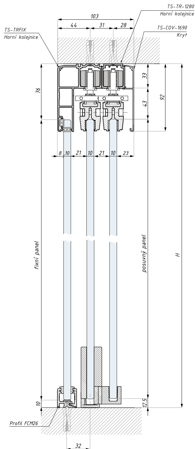
Montáž do stropu
