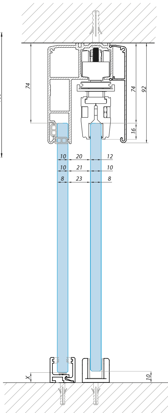
Montaż do sufitu z panelem stałym
