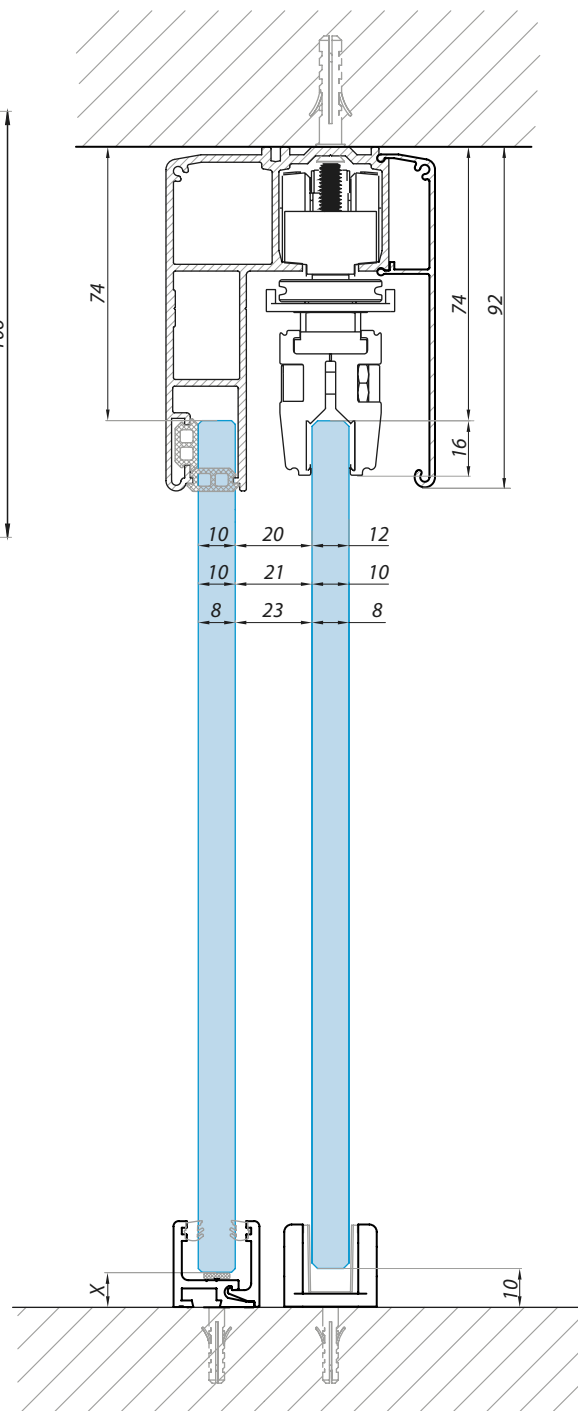
Montaż do sufitu z panelem statym
