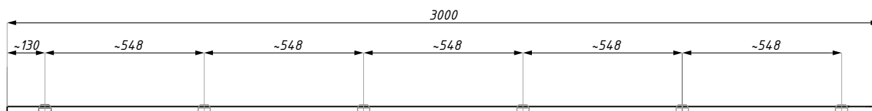
Zalecane rozmieszczenie oraz ilość elementów kotwiących
