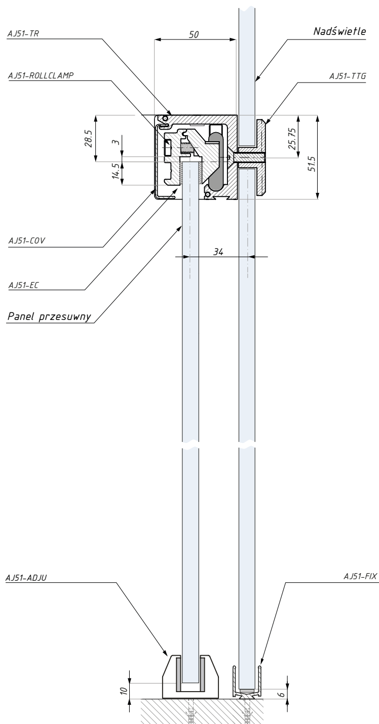
Montaż do szkła (nadświetle + boczne panele statel)
