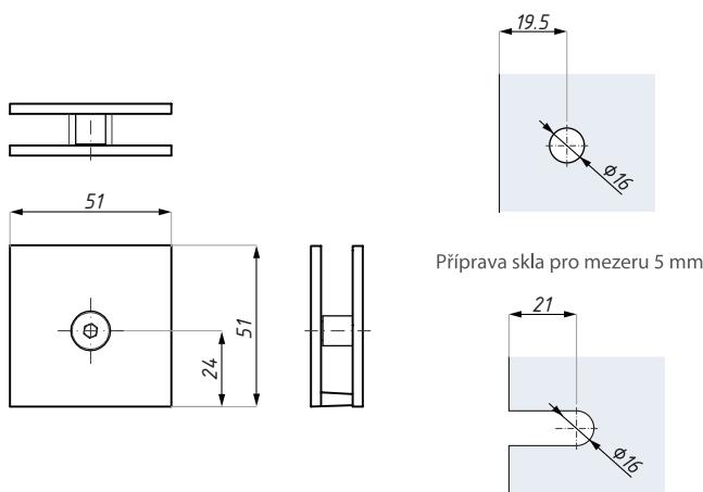
Příprava skla pro mezeru 0-5 mm
