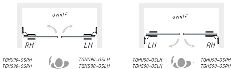
Závěsy (zed' - sklo), boční montáž
