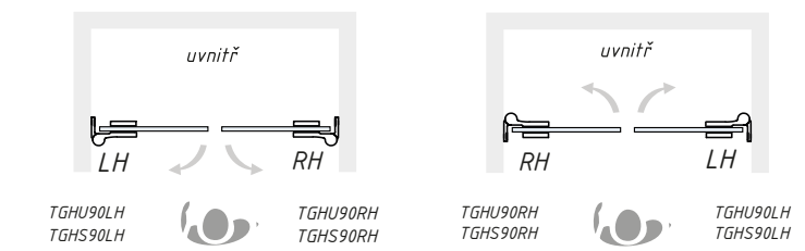
Závěsy (zed' - sklo)
